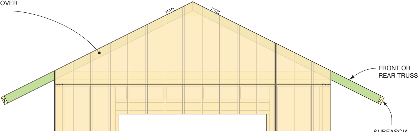
VIEW A-A
